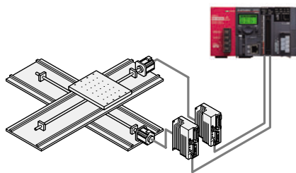
Подключение двух сервоосей непосредственно к процессорному модулю контроллера
