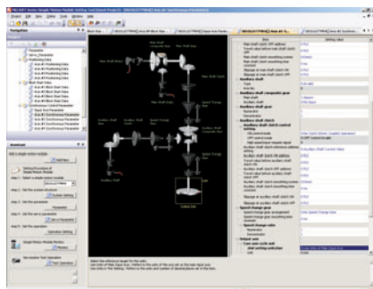
Окно параметров синхронного управления
