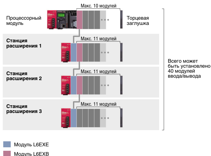
Расширение системы с процессорным модулем L26CPU-PBT при помощи модулей L6EXB/L6EXE
