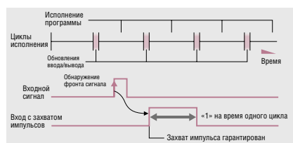
Функция захвата коротких импульсов
