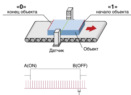
Измерение длины объекта при помощи функции измерения длительности импульсов
